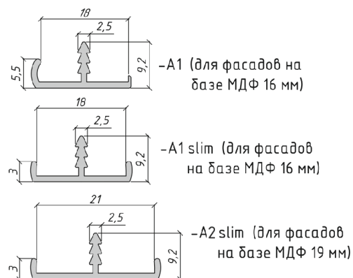
Виды аллюминиевого профиля с основными техническими параметрами
