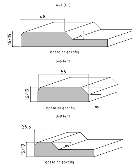
Возможный вариант профиля фрезы "по фасаду"
