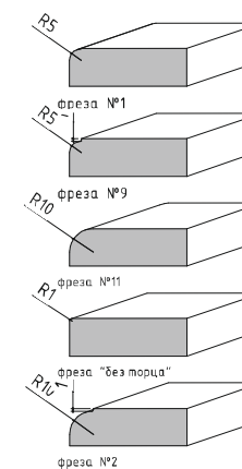
Возможный вариант профиля «по торцу»
