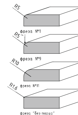
Возможный вариант профиля «по торцу»
