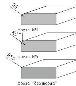
фреза "без торца"
