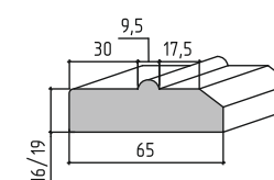
С-С (3:1)
