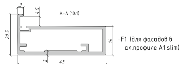
Виды аллюминиевых профилей для изготовления рамок с основными техническими параметрами
