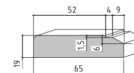
C-C (3:1)
