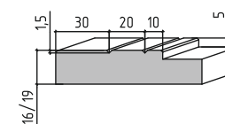
B-B (3:1)
