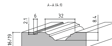
Возможный вариант профиля «по фасаду»
