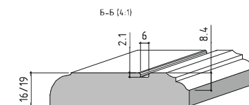
Возможный вариант профиля «по торцу»
