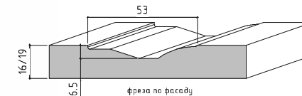
Возможный вариант профиля «по фасаду»
