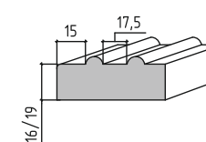
С-С (3:1)
